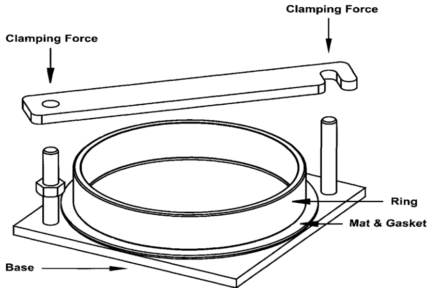
Fig. 1. Specimen holder.
